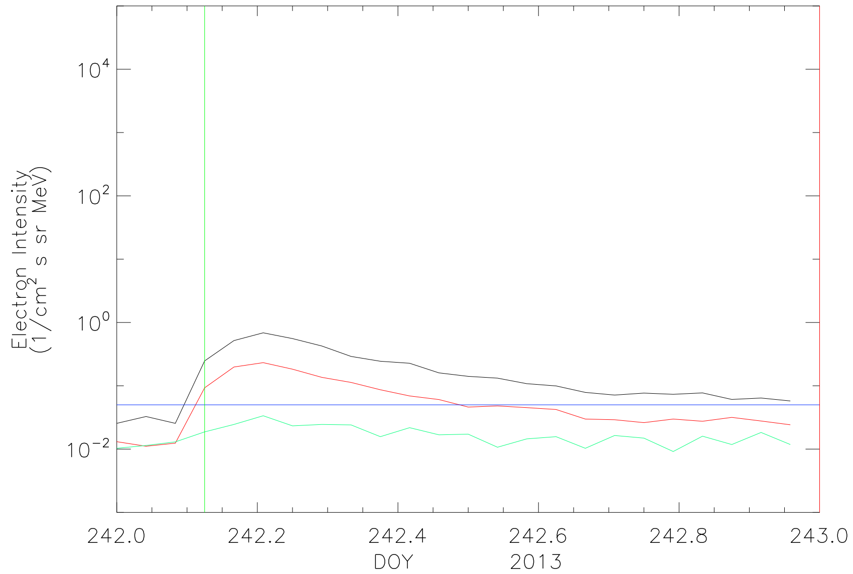
STEREO Behind HET Electron Data HET_electrons_2013.660645.pdf
