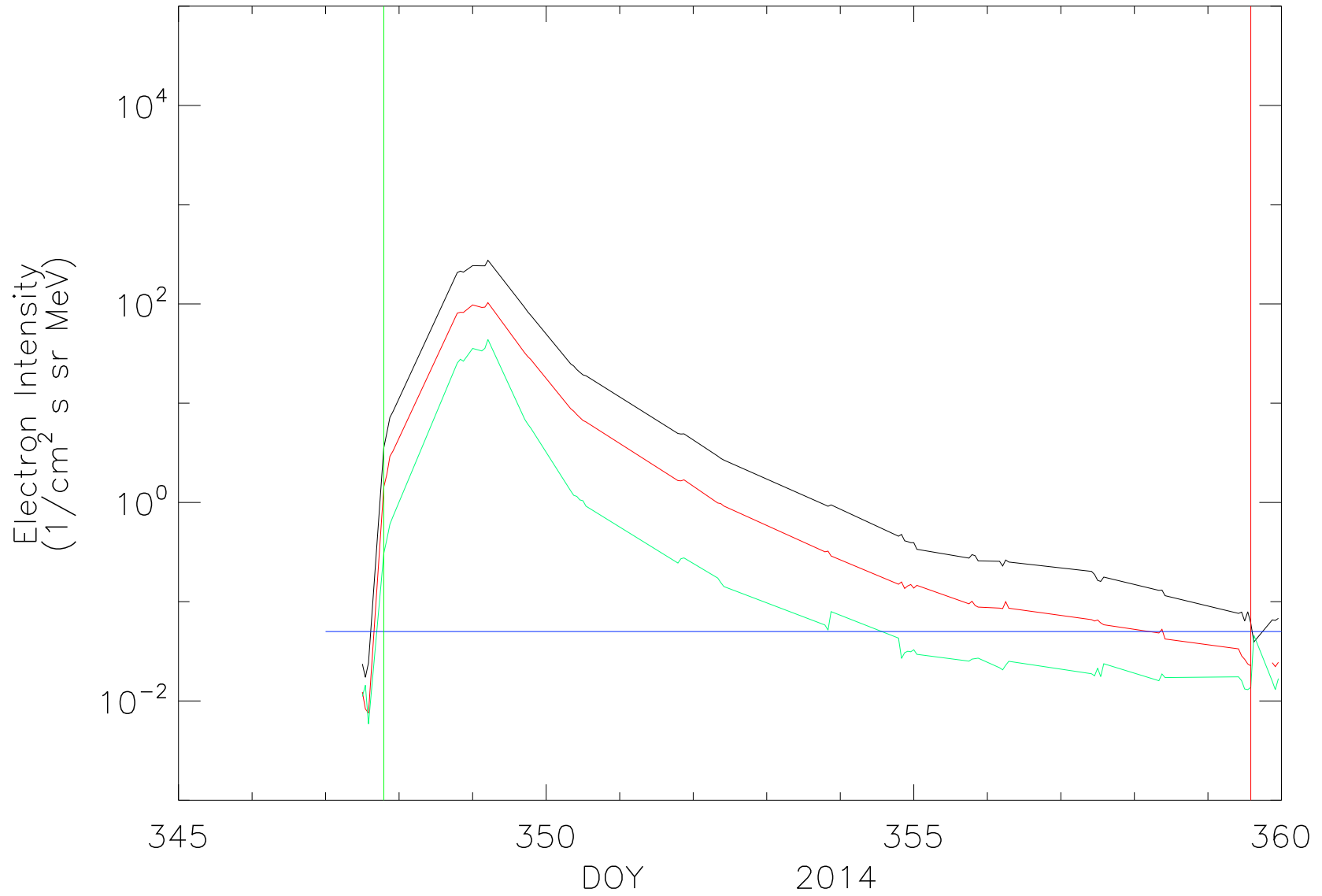
STEREO Ahead HET Electron Data HET_electrons_2014.950073.pdf
