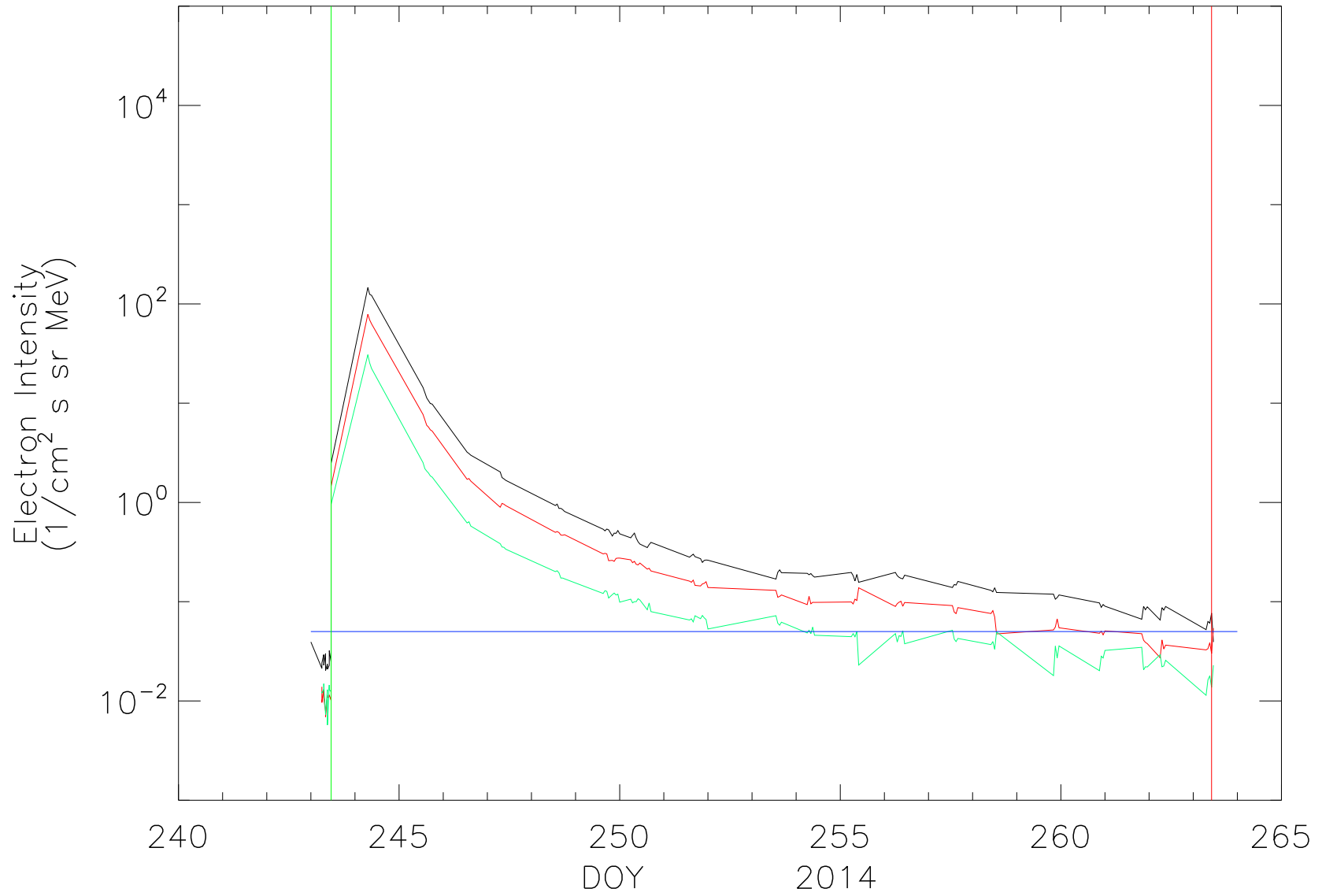
STEREO Ahead HET Electron Data HET_electrons_2014.664307.pdf
