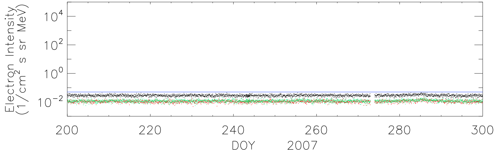
STEREO Ahead HET Electron Data
